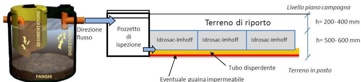
Figura 2. Schema di depurazione e smaltimento delle acque reflue tramite sistema IDROSAC IMHOFF
