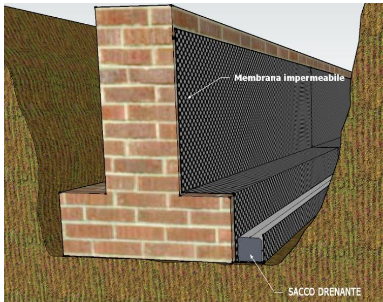
Fig.8. Sezione tipo. Applicazione sacco drenante con membrana impermeabile a protezione della fondazione.
