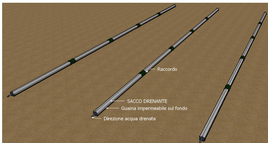
Fig.9. Configurazione parallela di sacchi drenanti 100.
